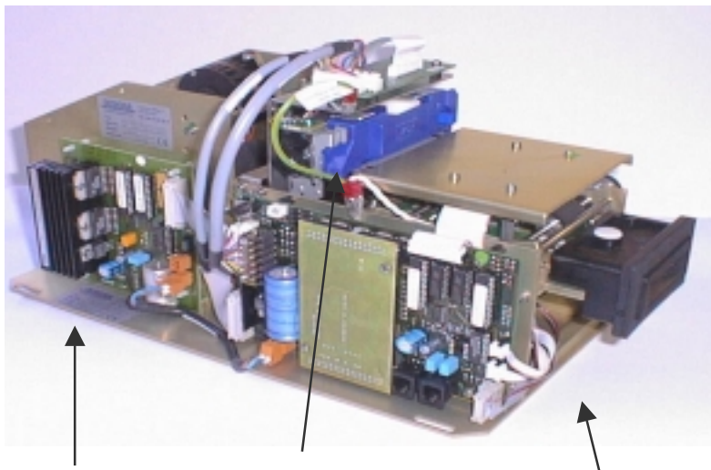
Transportbaugruppe TBG transport unit TBG Nadelrucker needle printer Magnetspureser / Grundgerät GG magnetic track reader / basic device GG
