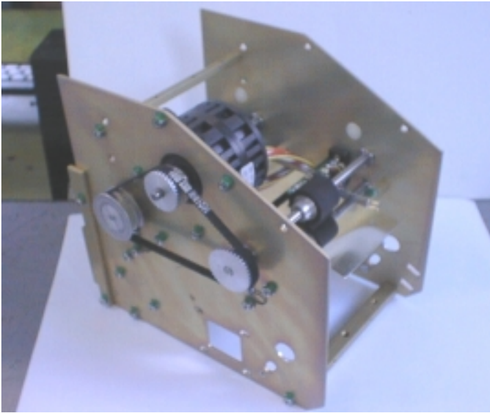
Transportbaugruppe 2 transport unit 2 2 780 411 693
