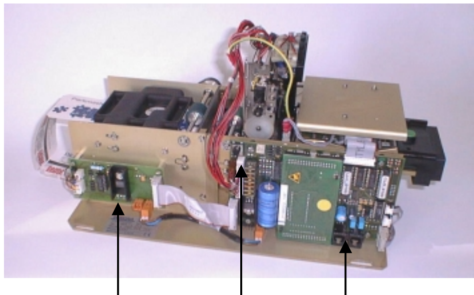
Transportbaugruppe transportation unit
